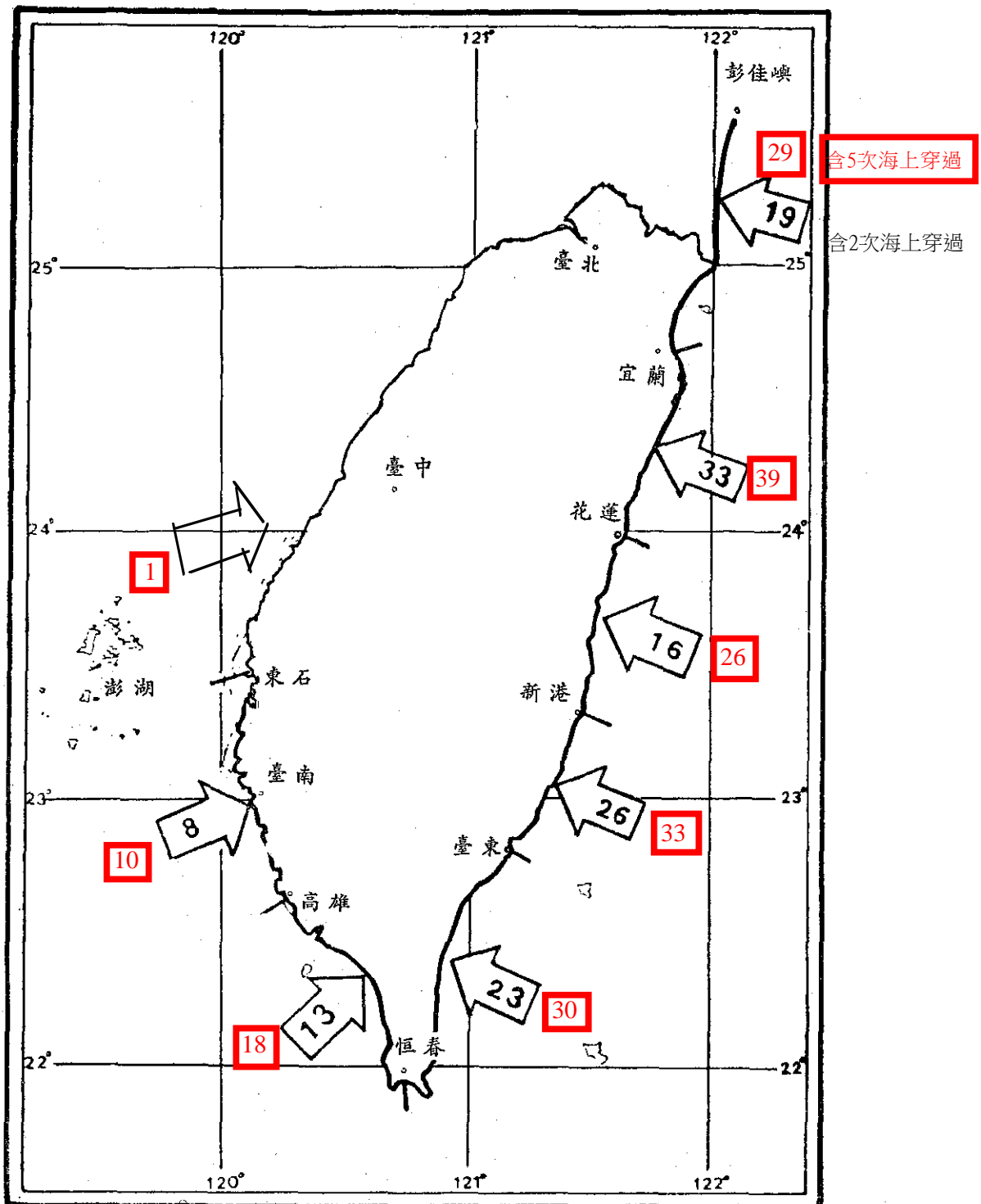
圖三十：颱風登陸地點之分段統計 (1897-1976)
