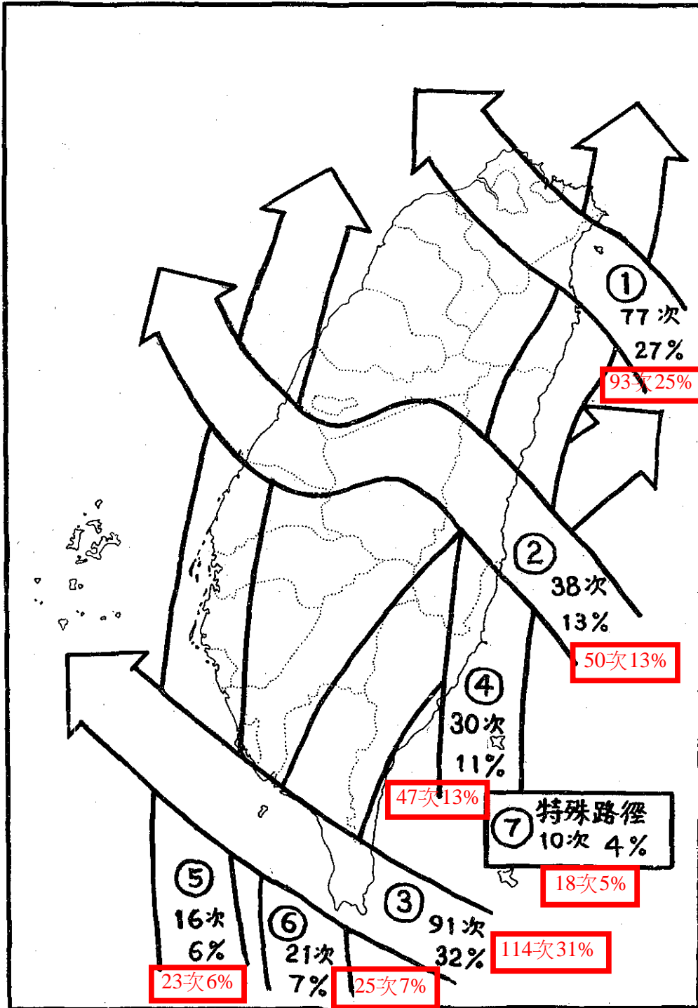
圖二十九：侵臺颱風路徑分類統計 (1897-1976)
