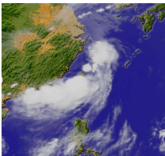
圖 13 敏督利颱風所引發西南氣流之衛星雲圖
