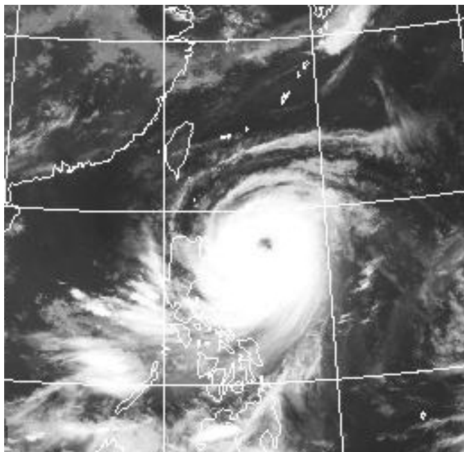
圖3 白色颱風環流中之黑點即為颱風眼
