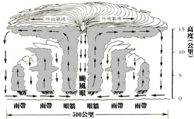
圖 2 颱風結構垂直剖面圖
