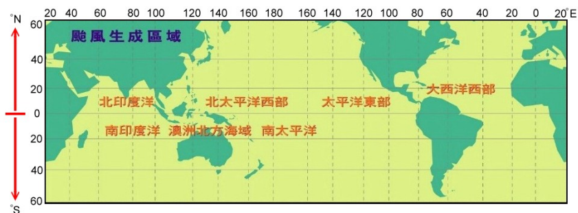
圖 1 颱風生成區域圖
