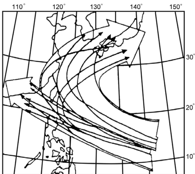
圖 5 北太平洋西部颱風路徑圖
