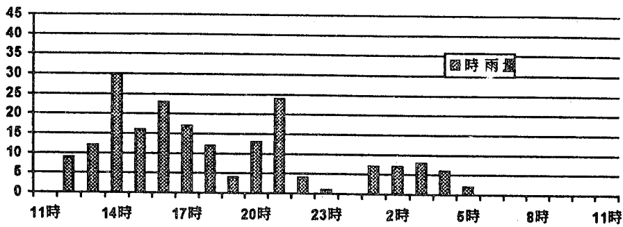
圖 6. 台東氣象站四日11時至五日11時期間逐時雨量圖(單位:mm)
