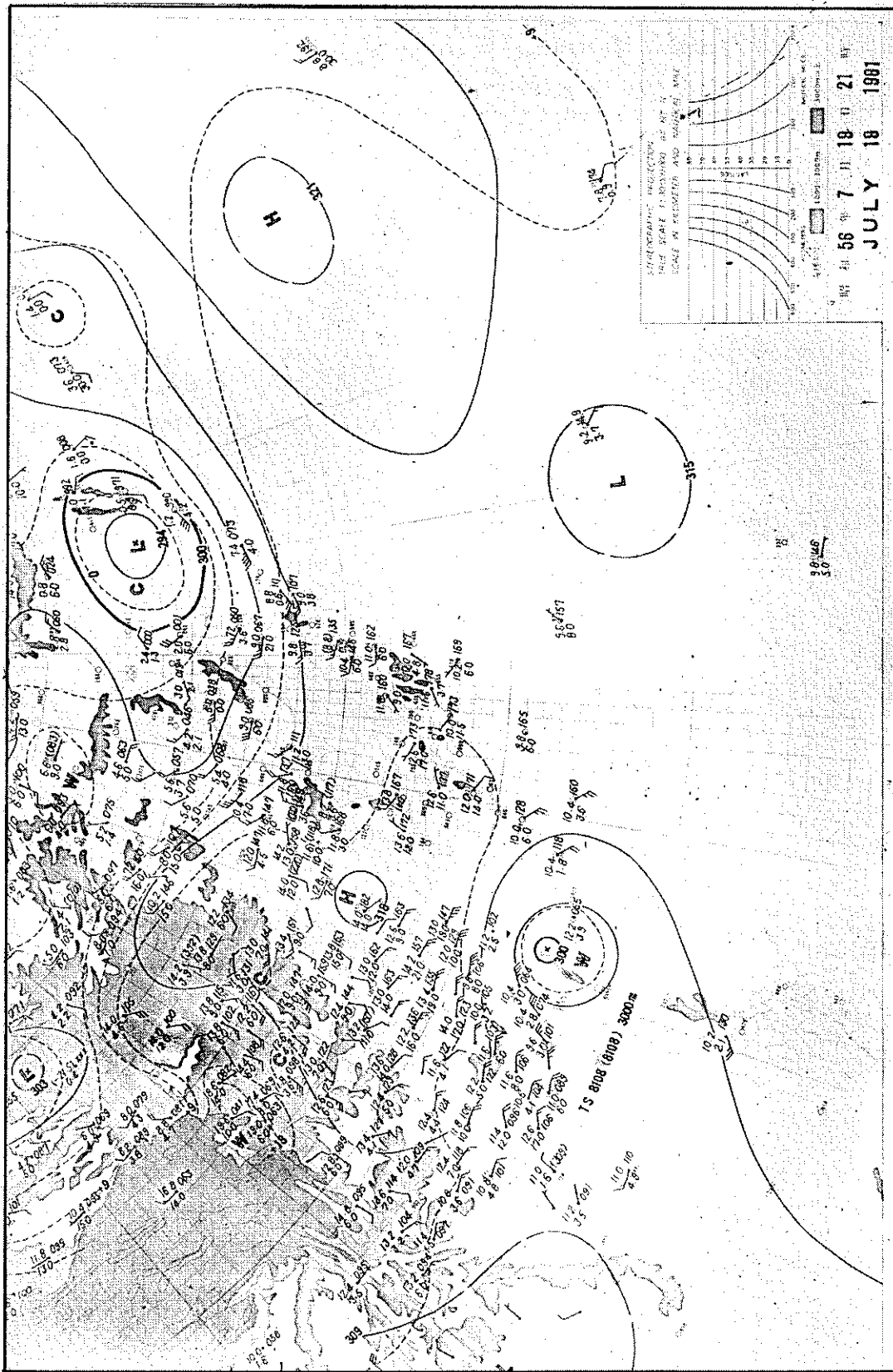
圖 3. 民國 70 年 7 月 19 日 00Z 700mb 高空圖 Fig. 3. 190000Z July 1981, 700mb chart
