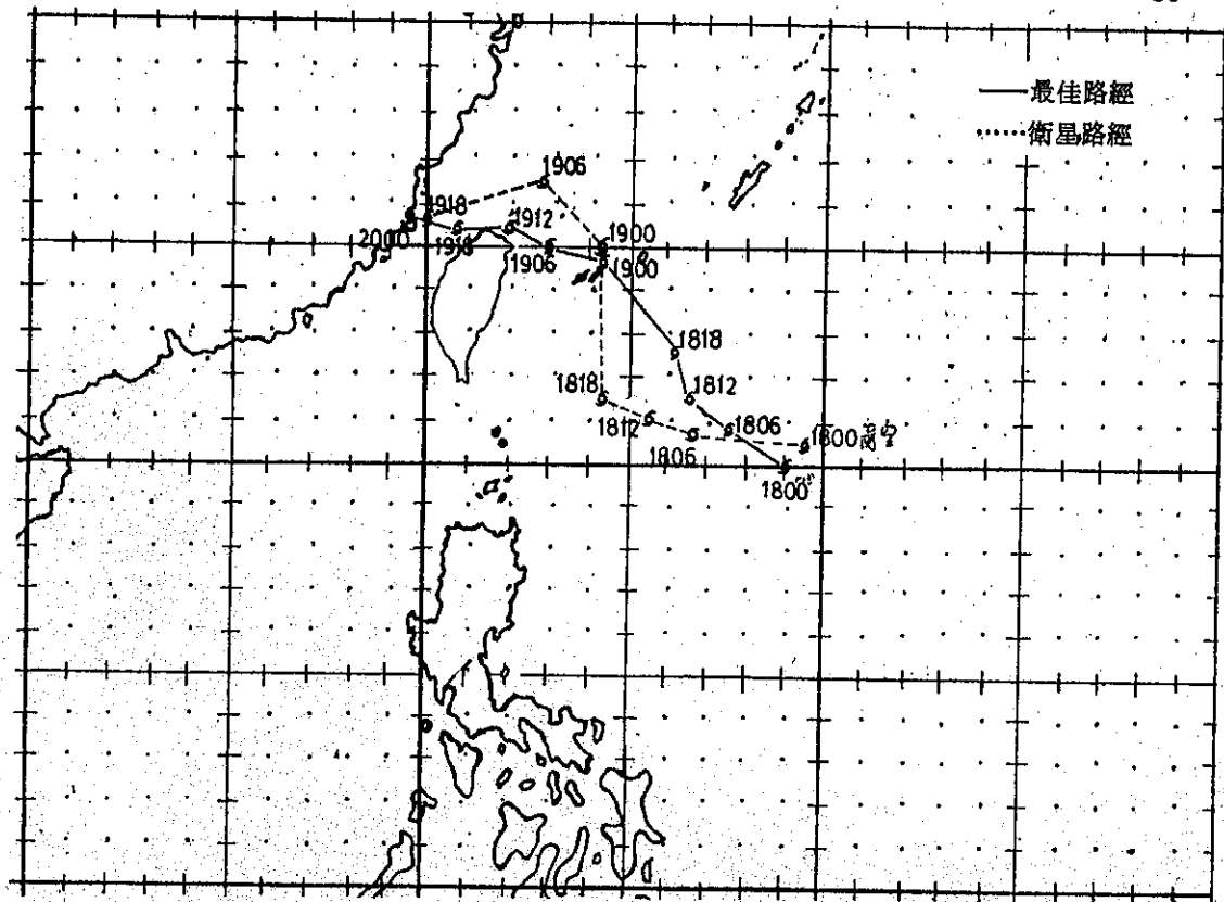
圖1. 莫瑞颱風路徑圖 Fig. 1. The best and satellite tracks for Typhoon Maury
