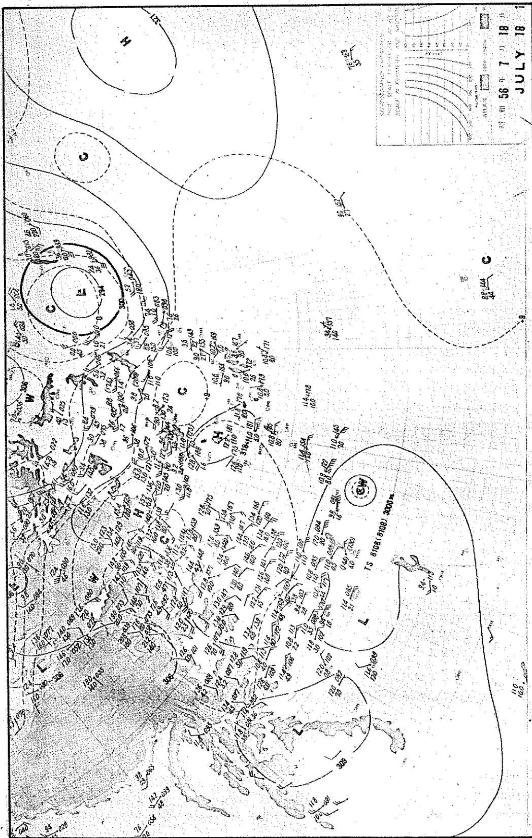
圖 2. 民國 70 年 7 月 18 日 12Z 700mb 高空圖 Fig. 2. 181200Z, July 1981, 700mb chart
