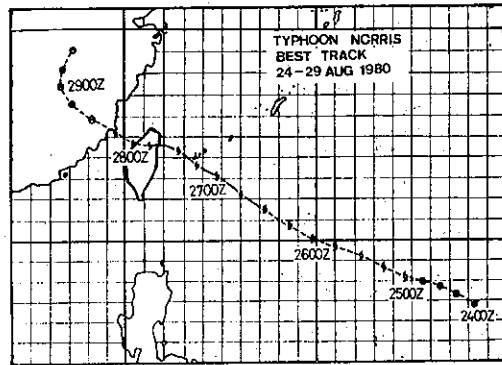
圖 12. 諾瑞斯颱風最佳路徑圖 Fig. 12 Best track of typhoon Norris (2400Z-2912Z Aug. 1980)
