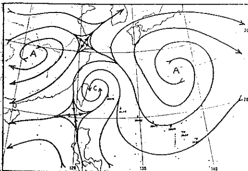
圖 8. 69年 8月 2712Z 三層 (700, 500, 300mb) 平均流線圖 Fig. 8. 3-level mean flow chart at 2712Z Aug. 1980.
