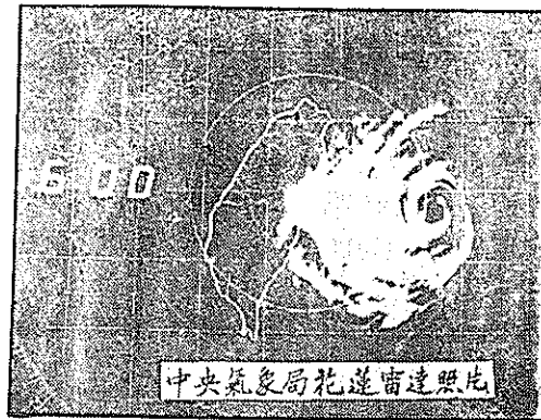
圖 10. 諾瑞斯颱風強度最強時期的雷達回波照片 Fig. 10. Hualien PPL radar picture at 2706Z Aug. 1980.
