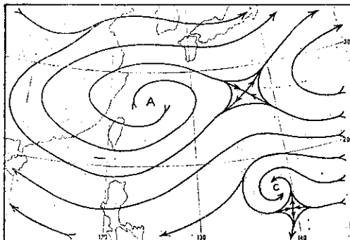
圖 3. 69年 8月 2400Z 三層 (700, 500, 300mb) 平均流線圖 Fig. 3 3-level mean flow chart at 2400Z Aug. 1980.
