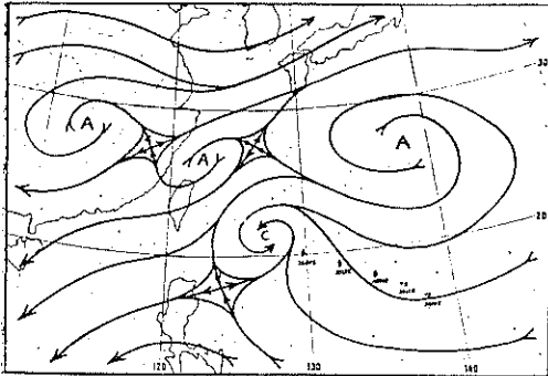
圖 6. 69年 8月 2612Z 三層 (700, 500, 300mb) 平均流線圖 Fig. 6. 3-level mean flow chart at 2612Z Aug. 1980.
