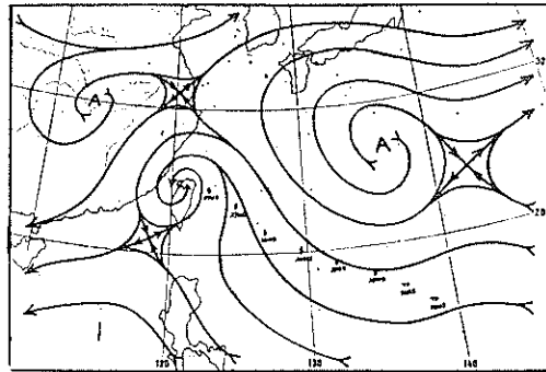
圖 9. 69年 8月 2800Z 三層 (700, 500, 300mb) 平均流線圖 Fig. 9. 3-level mean flow chart at 2800Z Aug. 1980.
