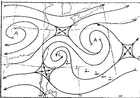
圖 7. 69年 8月 2700Z 三層 (700, 500, 300mb) 平均流線圖 Fig. 7. 3-level mean flow chart at 2700Z Aug. 1980.
