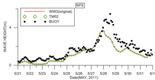
圖10 修正前後的波高與實測波高比較時序列圖-以NFS風場模擬波浪
