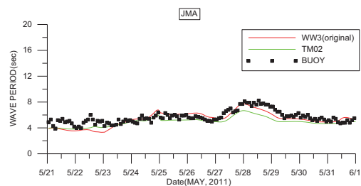
圖3 修正前後的周期與實測周期比較時序列圖-以JMA風場模擬波浪
