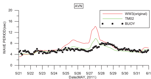
圖2 修正前後的周期與實測周期比較時序列圖-以AVN風場模擬波浪
