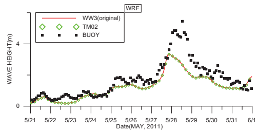
圖11 修正前後的波高與實測波高比較時序列圖-以WRF風場模擬波浪
