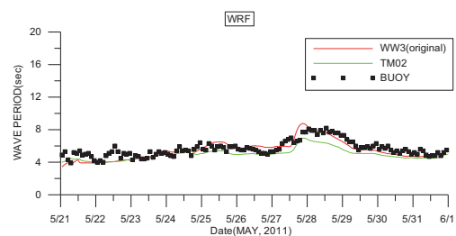
圖5 修正前後的周期與實測周期比較時序列圖-以WRF風場模擬波浪
