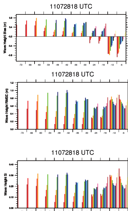
圖15 過去72小時波高的實測資料與預報資料誤差分析圖範例
