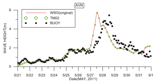
圖8 修正前後的波高與實測波高比較時序列圖-以AVN風場模擬波浪
