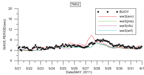
圖7 修正後的周期與實測周期比較時序列圖
