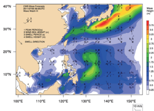
圖12 波浪等值圖範例
