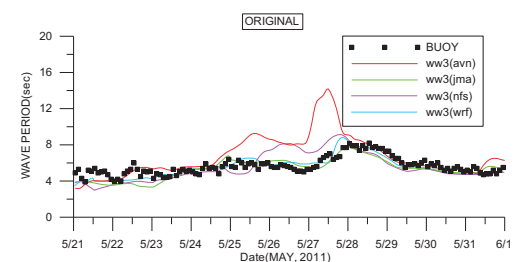
圖6 修正前的周期與實測周期比較時序列圖
