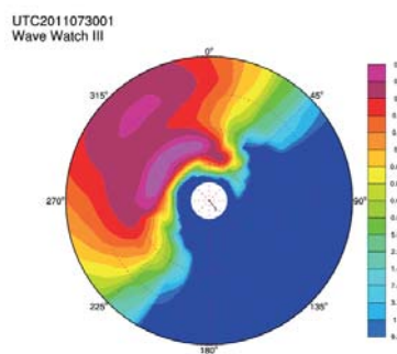
圖13 方向波譜圖範例
