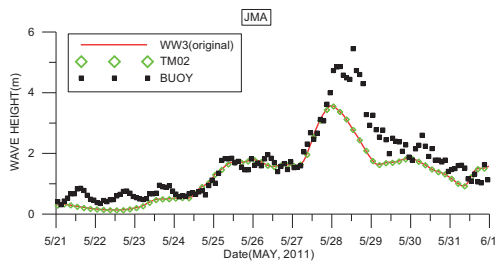
圖9 修正前後的波高與實測波高比較時序列圖-以JMA風場模擬波浪
