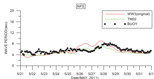
圖4 修正前後的周期與實測周期比較時序列圖-以NFS風場模擬波浪
