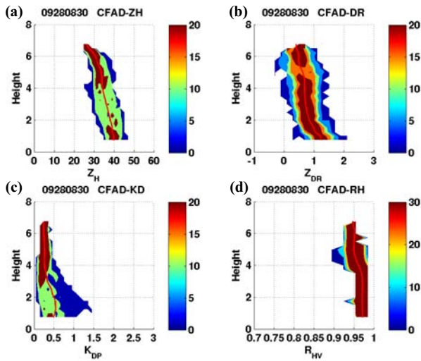
圖11 同圖10，『B點』觀測資料時間為2008年9月 28日0830 UTC。
