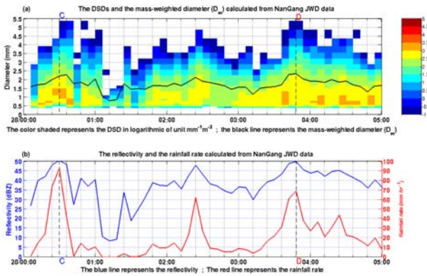
圖12 (a)為南港雨滴譜儀觀測雨滴粒徑分佈之時間 序列圖，縱軸表示雨滴等效體積直徑；色階部 份表示 N(D)(\text{mm}^{-1}\text{m}^{-3}) 值取對數( \log_{10} )，黑色實 線表示 D_m (mm)值。(b)為南港雨滴譜儀觀測資 料計算降雨率及反射率之時間序列圖，藍線為 反射率(dBZ)，紅線為降雨率( \text{mm hr}^{-1} )，左邊 縱軸表示反射率，右邊縱軸表示降雨率。(a)、 (b)橫軸表示時間序列(UTC)。
