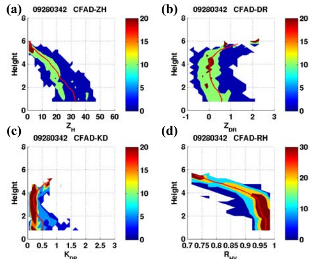
圖14 同圖10，『D點』觀測資料時間為2008年9月 28日0342 UTC。
