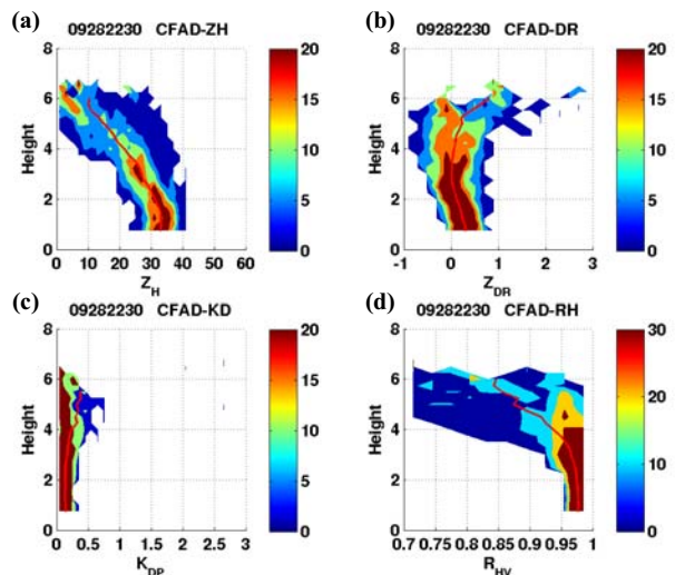
圖10 『A點』南港上空 10 \times 10 公里CFAD圖，(a)-(d)分別為 Z_H 、 Z_{DR} 、 K_{DP} 、RH(相關係數)圖，橫軸表示各參數值，縱軸表示高度，紅線為高
