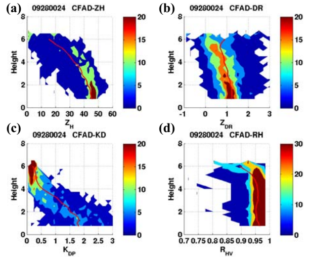
圖13 同圖10，『C點』觀測資料時間為2008年9月 28日0024 UTC。
