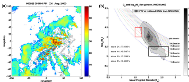
圖7 (a)2008年9月28日0034 UTC雷達 2.0^\circ 仰角PPI回波圖，黑色方框為反演DSD範圍；(b)機率密度分佈圖(PDF)，為(a)方框範圍反演結果，灰階部分代表分佈百分比。
