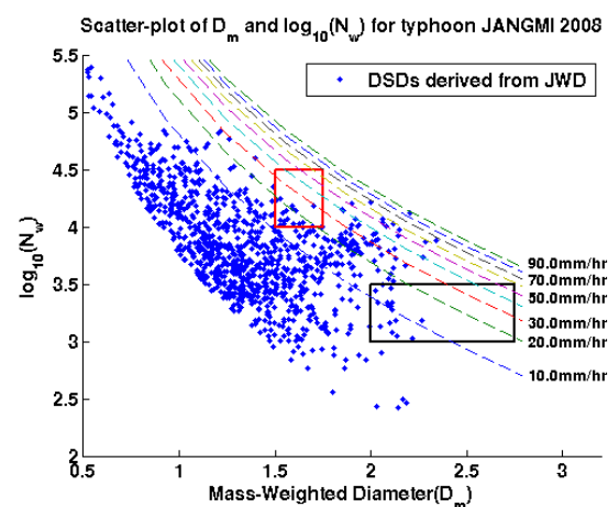
圖4 雨滴個數取對數( \log_{10}N_w )與 D_m 散佈關係圖，橫軸表示 D_m 值，縱軸表示 \log_{10}N_w 值，紅（黑）色方框表示海洋（大陸）型對流降雨系統，虛線表示降雨率，間隔為 10 \text{ mm hr}^{-1} 。
