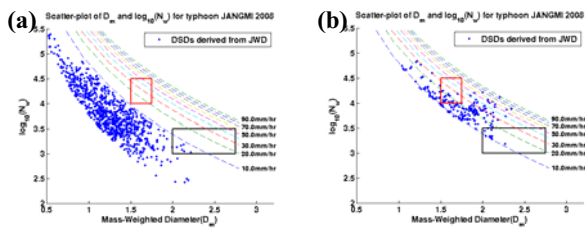
圖5 同圖4，(a)層狀降雨系統散佈圖，(b)對流降雨系統散佈圖。
