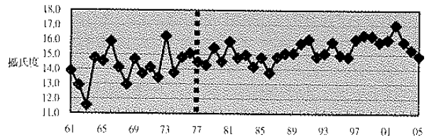
1961-2005 逐年 1-4 月每日最低溫度平均
