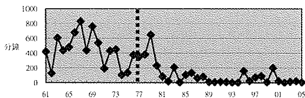
圖 5 台北松山機場 1961~2005 年 1~4 月能見度低於 800m 之發生時間(分鐘)分布
