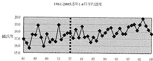
圖 2 台北松山機場 1961~2005 年 1~4 月逐年每月平均溫度分布
