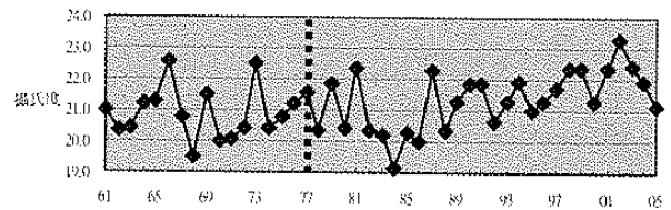
1961-2005 逐年 1-4 月每日最高溫度平均
