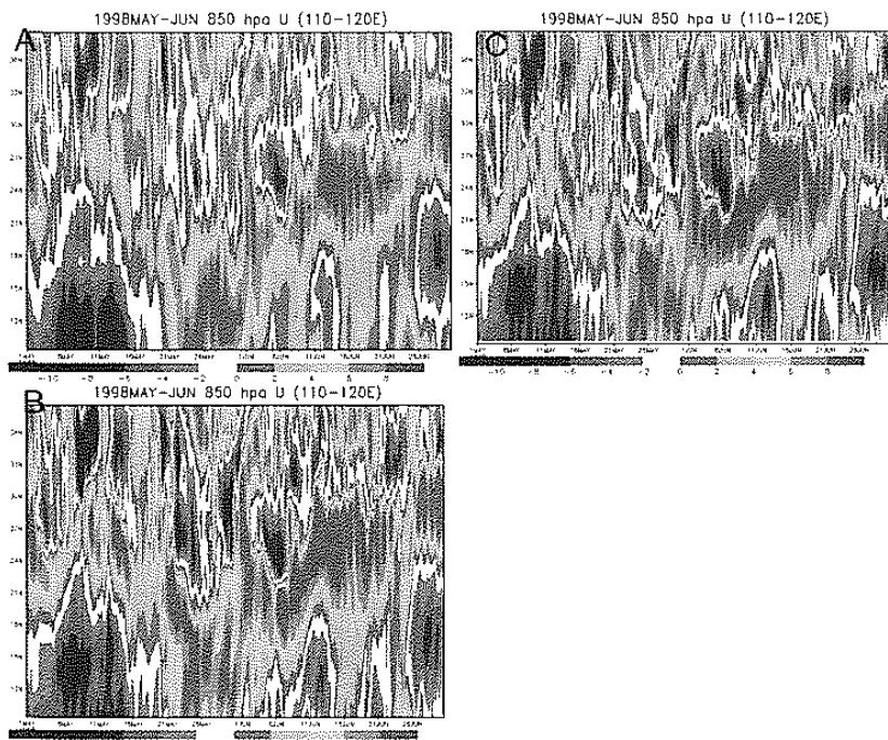
圖二 1998 年五至六月 110-120°E 區域平均緯向風場的緯度-時間剖面圖 (A) ERA40, (B) 60km 解析度, (C) 15km 解析度。
