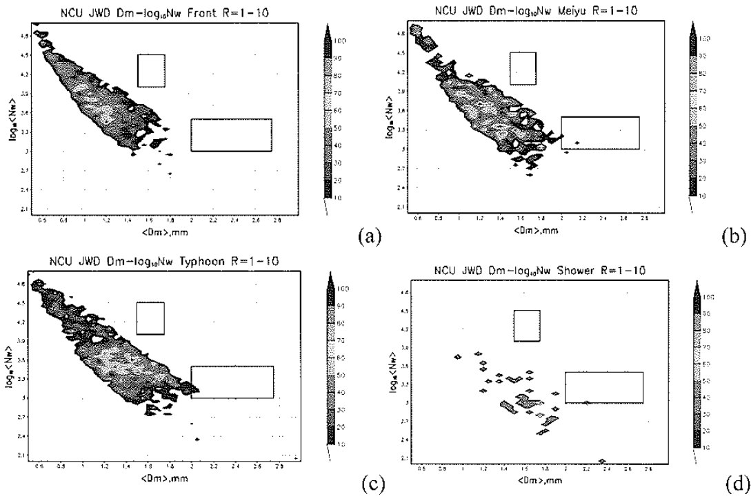
圖 2 分降水型態中央站 JWD 降雨率小於 10(mm/hr)之 D_m -log 10 ( N_w )散布圖。(a)為鋒面，(b)為梅雨，(c)為颱風，(d)為午後雷陣雨；橫軸代表 D_m ，縱軸代表次數 \log_{10}(N_w) ，不同色代表出現的機率。
