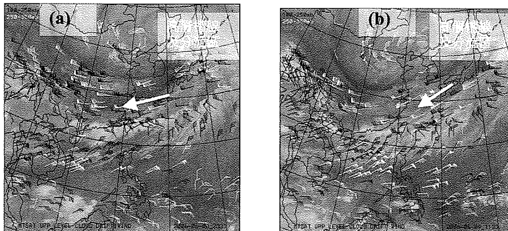
圖 3.2 2006 年 6 月 9 日 MTSAT-1R 東亞地區高層(500-100hPa)衛星風場，(a) 00UTC、(b) 12UTC。
