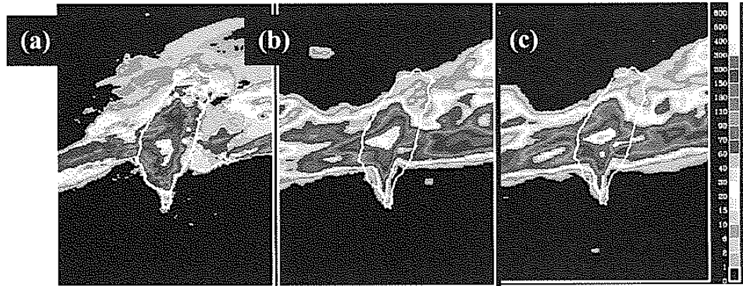
圖 3.3 LAPS-MM5 對 2006 年 6 月 9 日 00UTC 之 0 至 12 小時台灣地區雨量預報圖, (a)雷達觀測之估計值、(b)未加入衛星風場、(c)已加入衛星風場。
