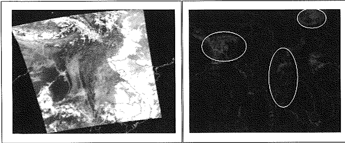
圖一、左圖為 MODIS/Aqua 東南亞 2004 年 3 月 4 日 06:45UTC 可見光圖，右圖為同一時間之煙塵偵測分布圖。
