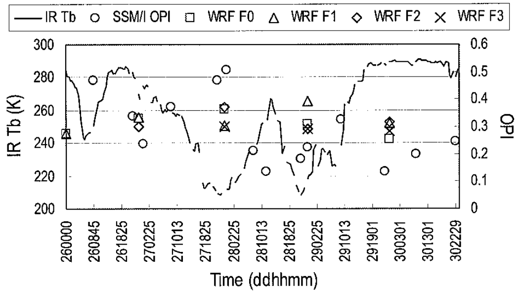
圖 5.6 IR 亮度溫度、SSM/I OPI, WRF OPI 初始分析場 (F0)、24 小時預報場 (F1)、48 小時預報場 (F2) 及 72 小時預報場 (F3) 時序變化圖。
