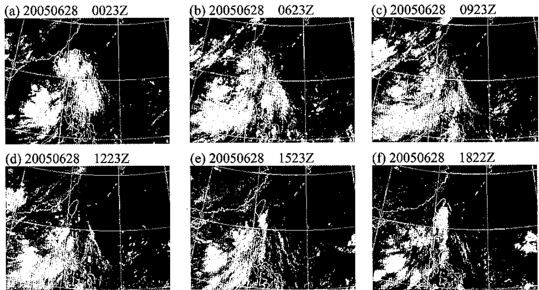
圖 5.5 2005 年 6 月 28 日 00 時至 6 月 28 日 21 時 22 分 GOES 9 紅外線衛星雲圖。
