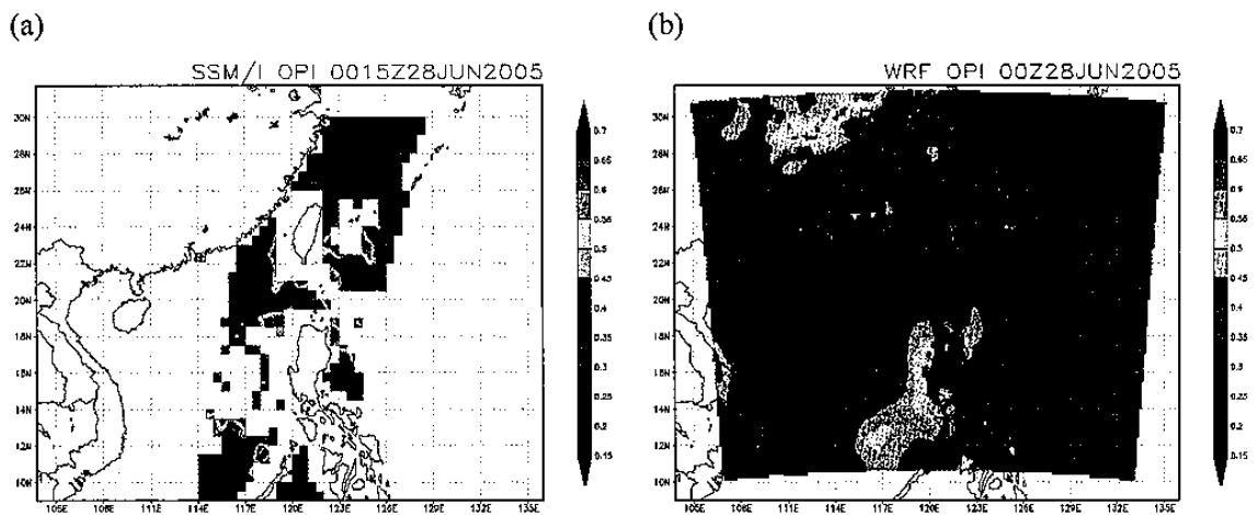
圖 5.4 (a) 2005 年 6 月 28 日 00 時 SSM/I OPI。(b)2005 年 6 月 28 日 00 時 WRF OPI。
