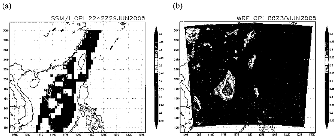
圖 5.1 (a) 2005 年 6 月 29 日 22 時 42 分 SSM/I OPI，(b) 2005 年 6 月 30 日 00 時 WRF OPI 初始分析場。
