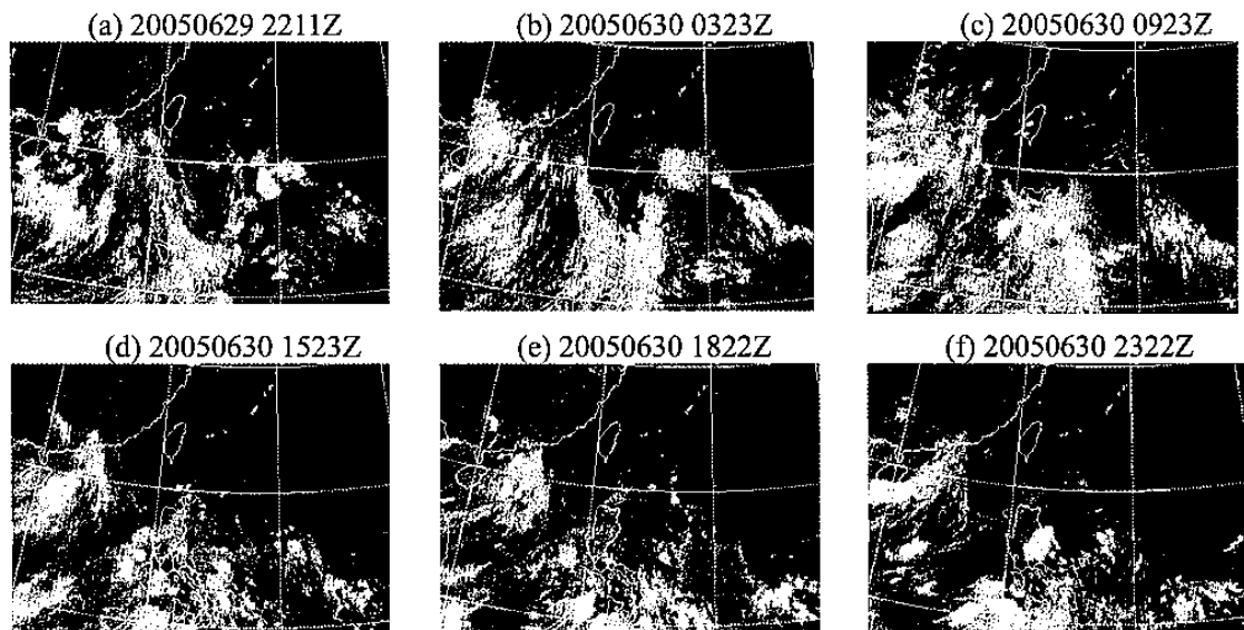
圖 5.2 2005 年 6 月 29 日 22 時至 6 月 30 日 23 時 GOES 9 紅外線衛星雲圖。
