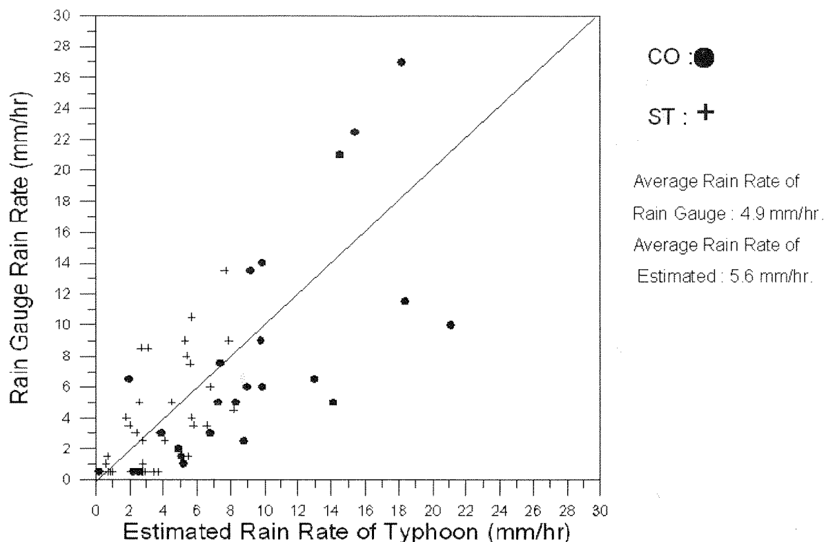
圖 2. 利用 2004 年於颱風期間 TMI 共計 66 筆資料對海上颱風降水強度迴歸式，進行與地面測站降雨真值做驗證，其兩者相關性達 0.74，均方根誤差為 3.75 mm/hr（CO 代表對流降水，ST 代表層狀降水）。
