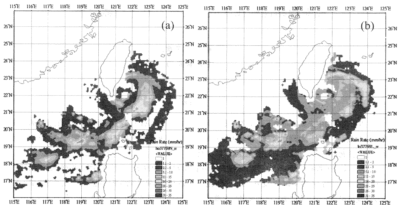
圖 4. 同圖 3.(a)為 2004/07/01 0448 UTC 敏督利颱風在接近本島利用 TMI 所估算出海上降水強度雨勢圖，(b) 為利用 Chen and Li 於梅雨期所建立之迴歸式求出海上降水強度分佈情形。
