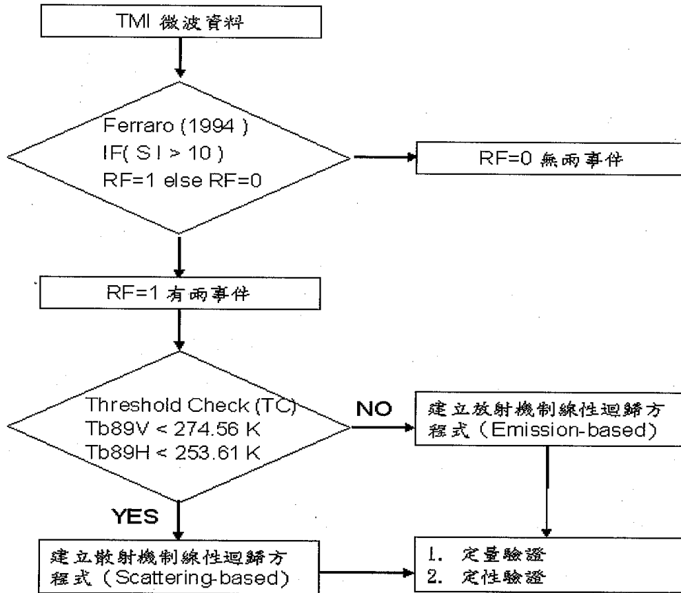
圖 1. 利用 TMI 微波資料反演海上颱風降水強度流程圖。
