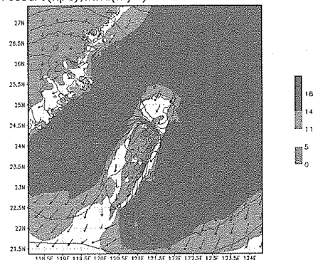
圖六 除去大陸東南丘陵地形。
