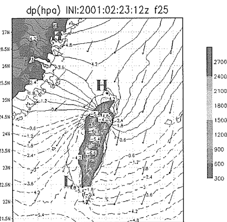
圖四 海平面氣壓變量分布。
