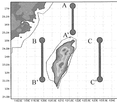
圖三 a 台灣北部海面、台灣海峽、台灣東部海面取剖面示意圖。
