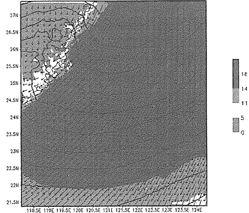
Pressure(hpa);Wind(m/s) INI:2001:02:23:12z f21
