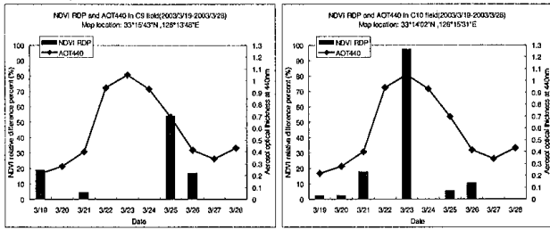
圖 5:濟州島測站之 AOT440 與附近 C1 至 C10 區域之 NDVI RDP 關係圖，資料時間：2003/3/19-2003/3/28，沙塵暴影響時間：2003/3/24-2003/3/26。
