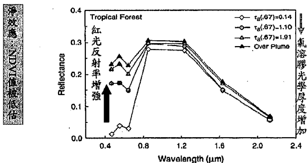
圖 1 MODIS 前五個頻道之反射率隨著光學厚度增加之情形。圖中 \tau_a(0.67) 表示 AERONET 測站所量得在 0.67 \mu\text{m} 的氣溶膠光學厚度 (Miura 等, 1998)。
