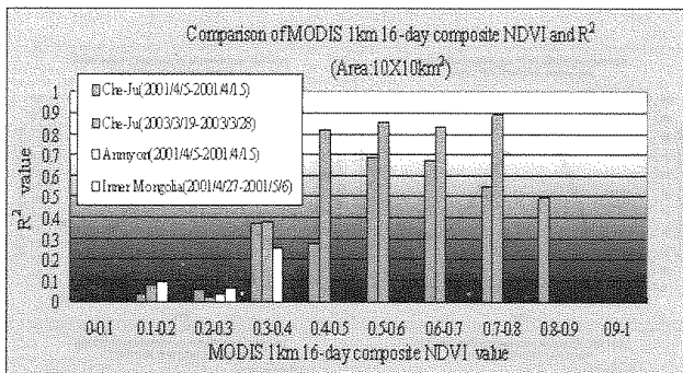
圖 2：不同背景值域與 AOT440 之相關性比較。Inner Mongolia 與 Anmyon 測站因其背景值域皆小於 0.4 故背景值域大於 0.4 時無資料。
