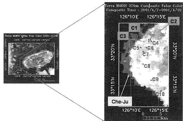
圖 3：在濟州島測站附近代號為 C1 至 C10 區域之位置。左圖為濟州島全島的真色影像 (True color image)，右圖為左圖區域放大之 16 日複合假色影像 (False color image)。
