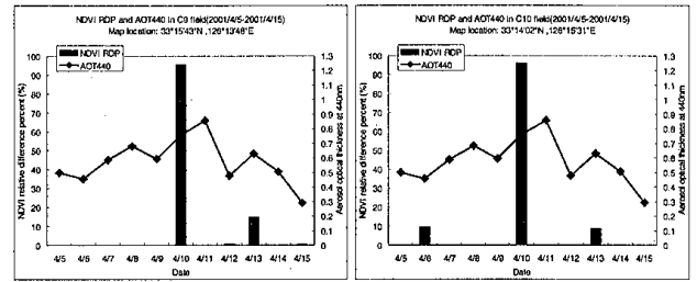
圖 4: 濟州島測站之 AOT440 與附近 C1 至 C10 區域之 NDVI RDP 關係圖，資料時間：2001/4/5-2001/4/15，沙塵暴影響時間：2001/4/7-2001/4/10。
