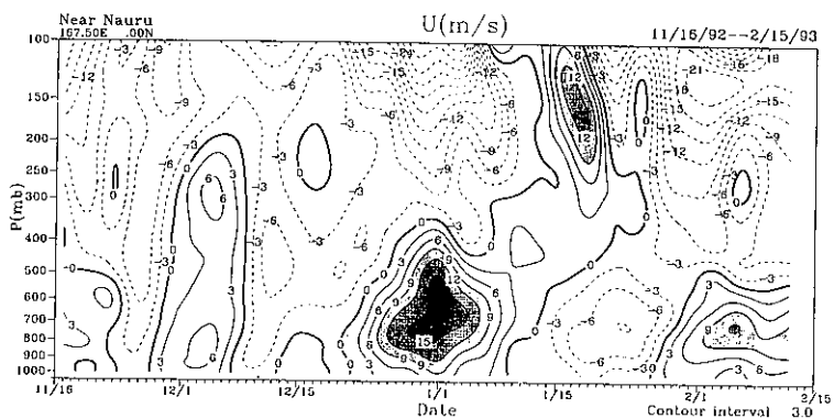
圖3 鄰近Nauru島格點的緯向風三天平均之垂直分佈時序。
