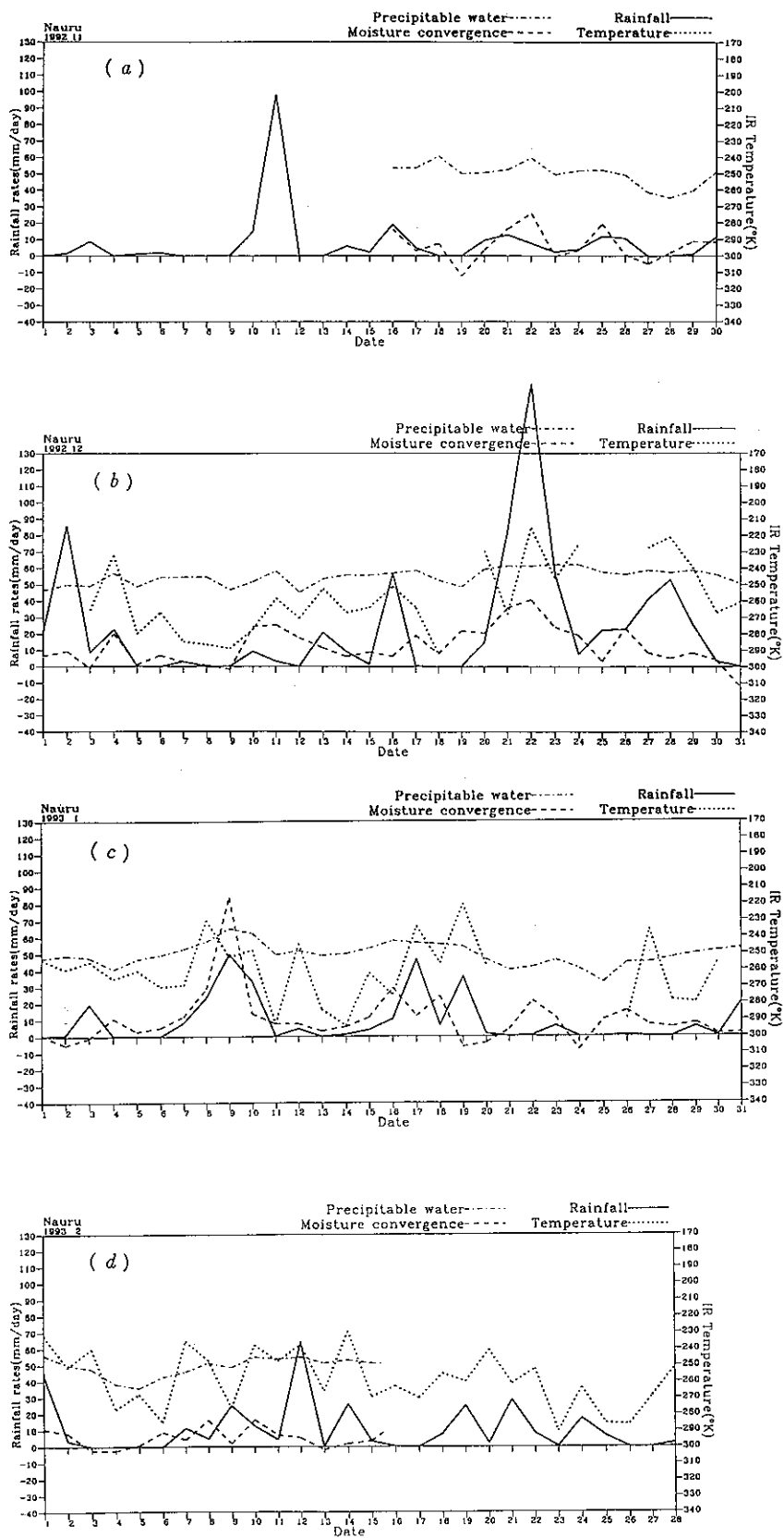
圖 18 Nauru 的可降水量、水汽輻合、雨量及 IR 溫度之時序。(a) 為 11 月，(b) 為 12 月，(c) 為 1 月，(d) 為 2 月。
