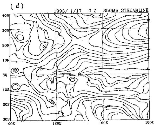
圖 17 西太平洋 850 hpa 流線場。(a) 11月18日，(b) 12月8日，(c) 1月1日， (d) 1月17日。
