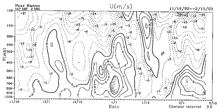
圖2 鄰近Manus島格點的緯向風三天平均之垂直分佈時序。
