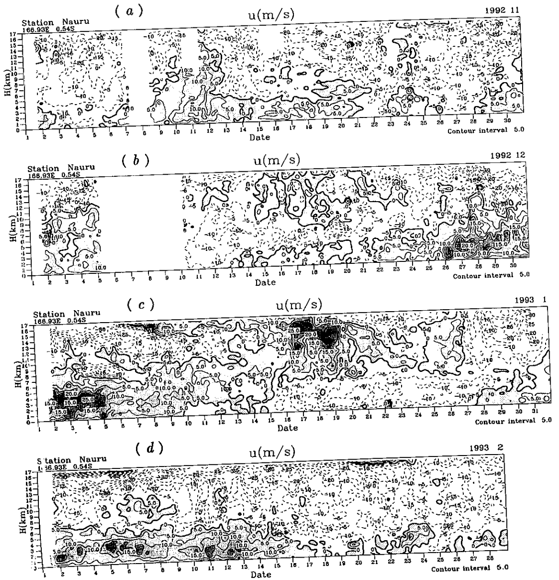
圖4 Nauru島探空所得緯向風之垂直時序。(a)為11月，(b)為12月，(c)為1月，(d)為2月。
