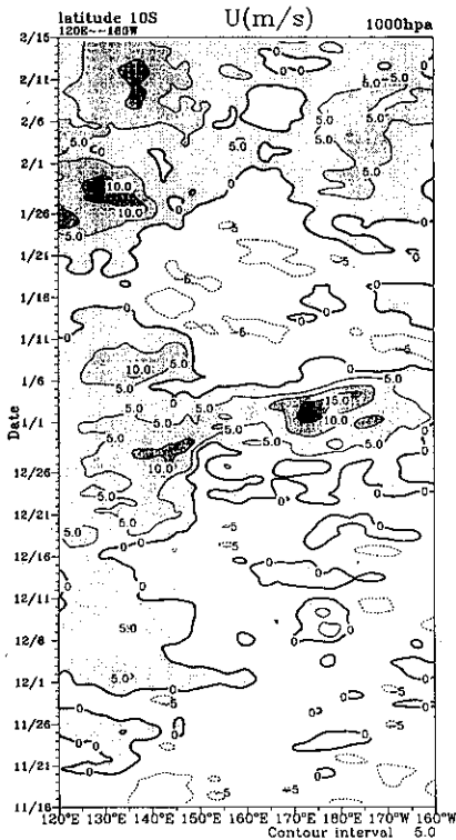
圖11 南緯10度，1000 hpa 緯向風日平均之緯向時序。
