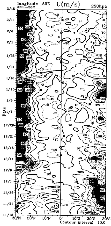
圖 13 東經 160 度，250 hpa 緯向風日平均之經向時序。
