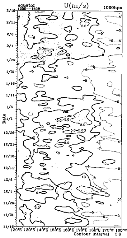
圖5 赤道1000 hpa緯向風日平均之緯向時序。
