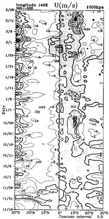
圖8 東經140度，1000 hpa緯向風日平均之經向時序。
