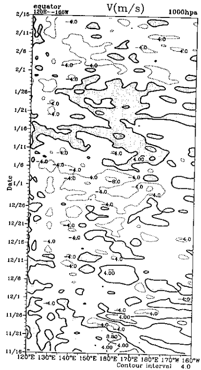
圖 16 赤道 1000 hpa 經向風日平均之緯向時序
