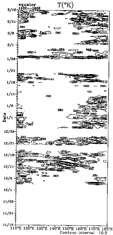
圖 15 赤道 IR 溫度半天平均之緯向時序。
