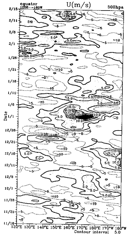
圖6 赤道500 hpa緯向風日平均之緯向時序。
