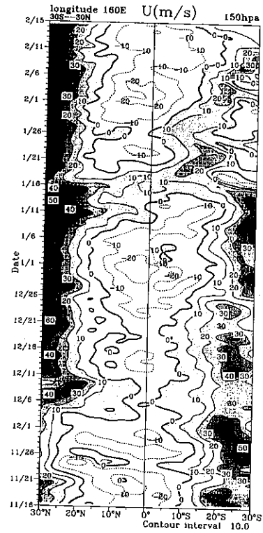
圖 14 東經 160 度，150 hpa 緯向風日平均之經向時序。
