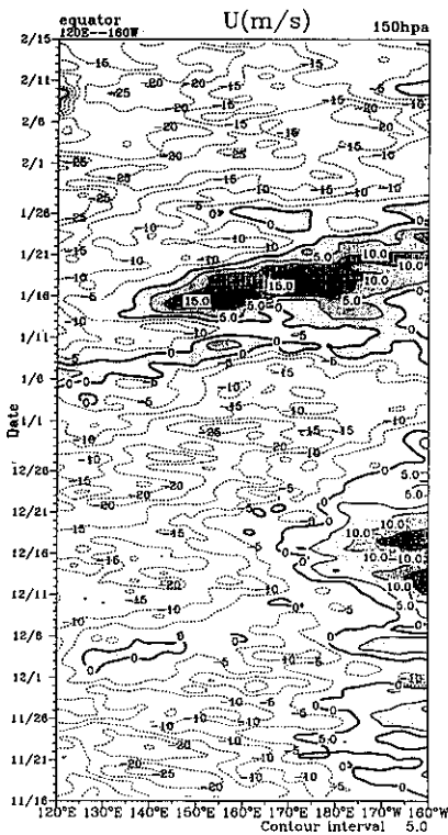
圖7 赤道150 hpa緯向風日平均之緯向時序。
