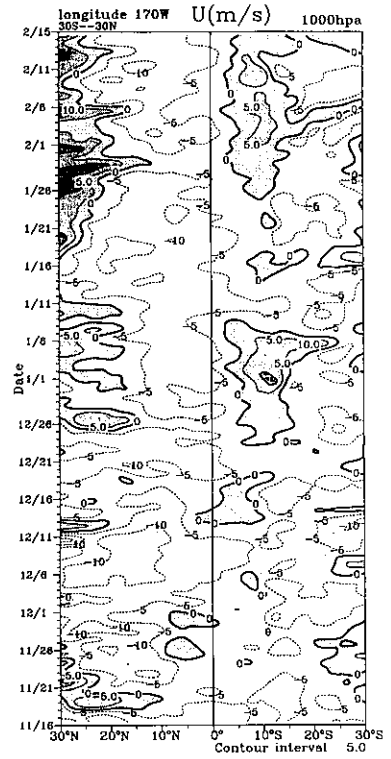
圖10 西經170度，1000 hpa 緯向風日平均之經向時序。
