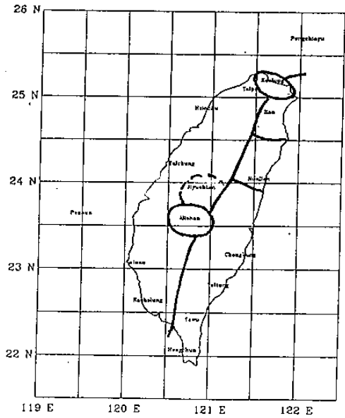
圖6：同圖 2，但爲秋季 ( a ) 九月 ( b ) 十月。
