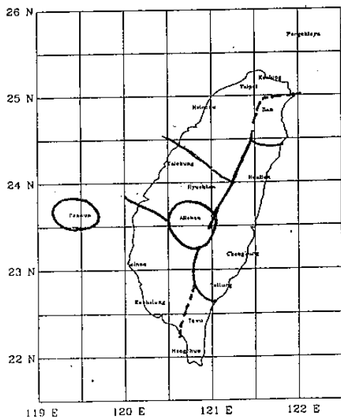
圖 4 : 同圖 2, 但為梅雨季 ( a ) 五月 ( b ) 六月。
