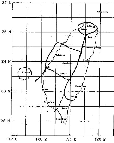
圖5：同圖 2，但爲仲夏 ( a ) 七月 ( b ) 八月。
