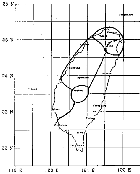
圖6：同圖 2，但爲秋季 ( a ) 九月 ( b ) 十月。
