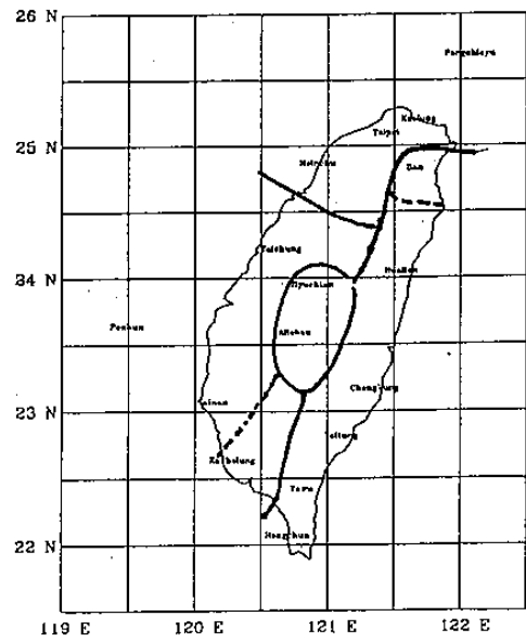
圖 3 : 同圖 2, 但為春季 ( a ) 三月 ( b ) 四月。
