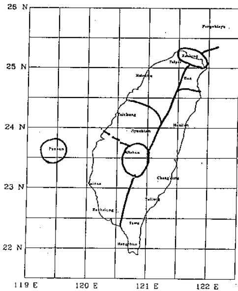
圖2：仲冬的氣候分區圖 ( a ) 一月 ( b ) 二月，實線表示氣候分區，虛線表示次區。
