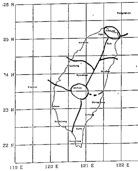
圖 8：台灣全年氣候分區圖，實線表示氣候分區，虛線表示次區。
