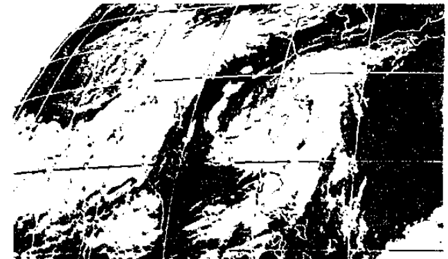
圖 1-14 1990年6月23日1200 UTC
