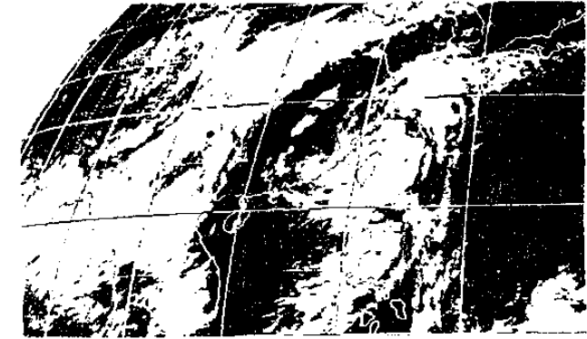
圖 1-15 1990年6月23日1500 UTC
