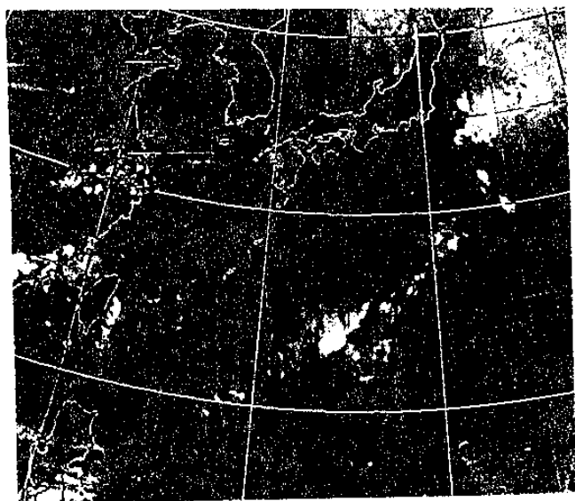
圖 3~5 1990年9月30日1800 UTC
