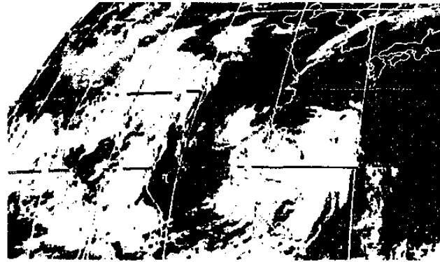
圖 1-10 1990年6月22日2100 UTC
