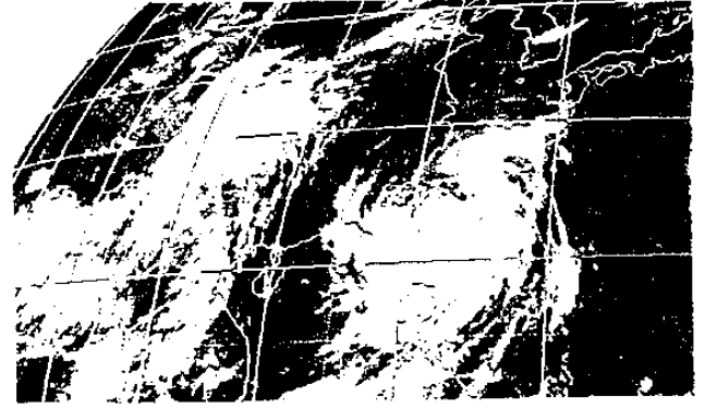
圖 1-12 1990年6月23日0300 UTC
