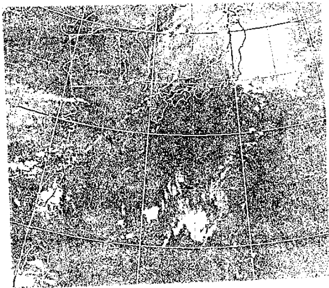
圖 3~4 1990年9月30日1200 UTC
