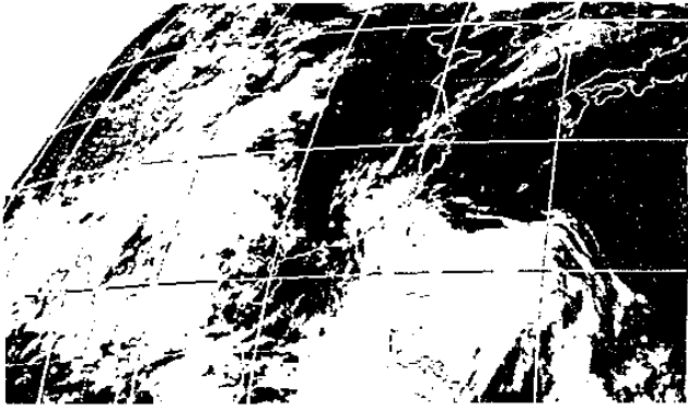
圖 1-8 1990年6月22日1200 UTC
