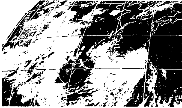
圖 1-9 1990年6月22日1800 UTC
