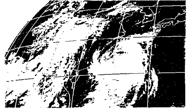
圖 1-13 1990年6月23日0600 UTC
