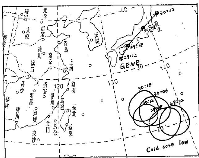
圖 4 1990年9月29~30日冷心低壓與傑恩颱風相對路徑圖。
