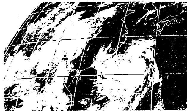
圖 1-11 1990年6月23日0000 UTC
