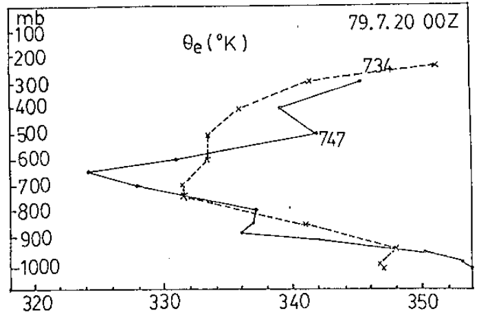
圖七：民國 79 年 7 月 20 日東港與馬公 00Z 相當
