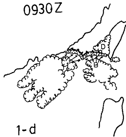
圖一-a 爲 0330 Z 觀測之可見光雲圖之分析；圖一-b 爲 0530 Z，圖一-c 爲 0830 Z；圖一-d 爲 0930 Z。
