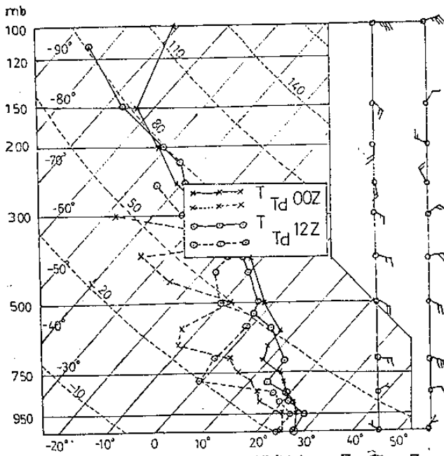
圖六：民國 79 年 7 月 20 日東港探空 00Z 與 12Z 之分析圖。
