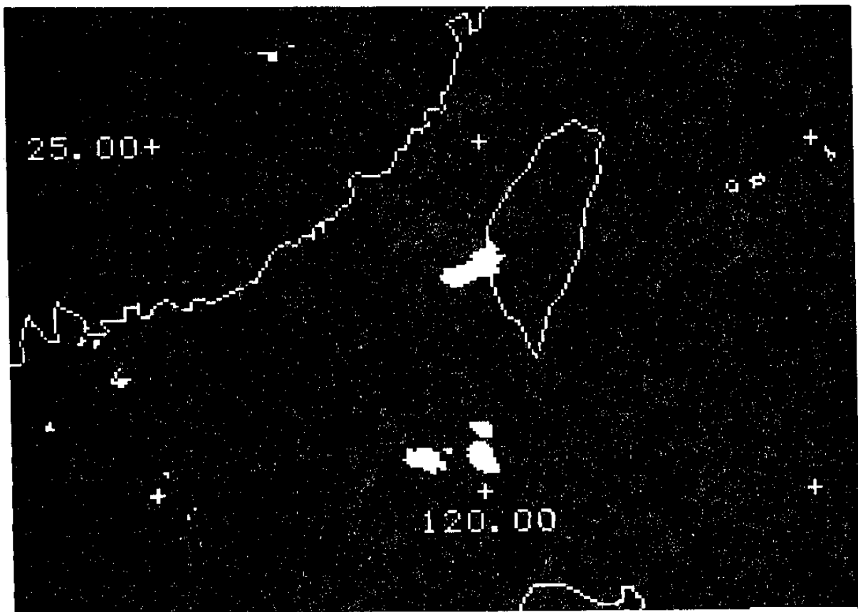
圖四：民國79年7月20日0933 Z GMS-04加強後之紅外線雲圖，加強曲綫使用MB-Curve。
