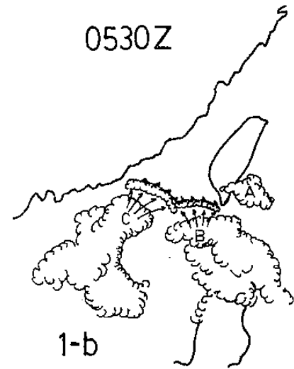
圖一：民國 79 年 7 月 20 日 GMS-04 可見光雲系分析圖，箭頭爲對流外流，弧狀雲綫前方之鋒面符號代表對流外流邊界，A, B, C, D, 分別代表主要的四個對流系統。
