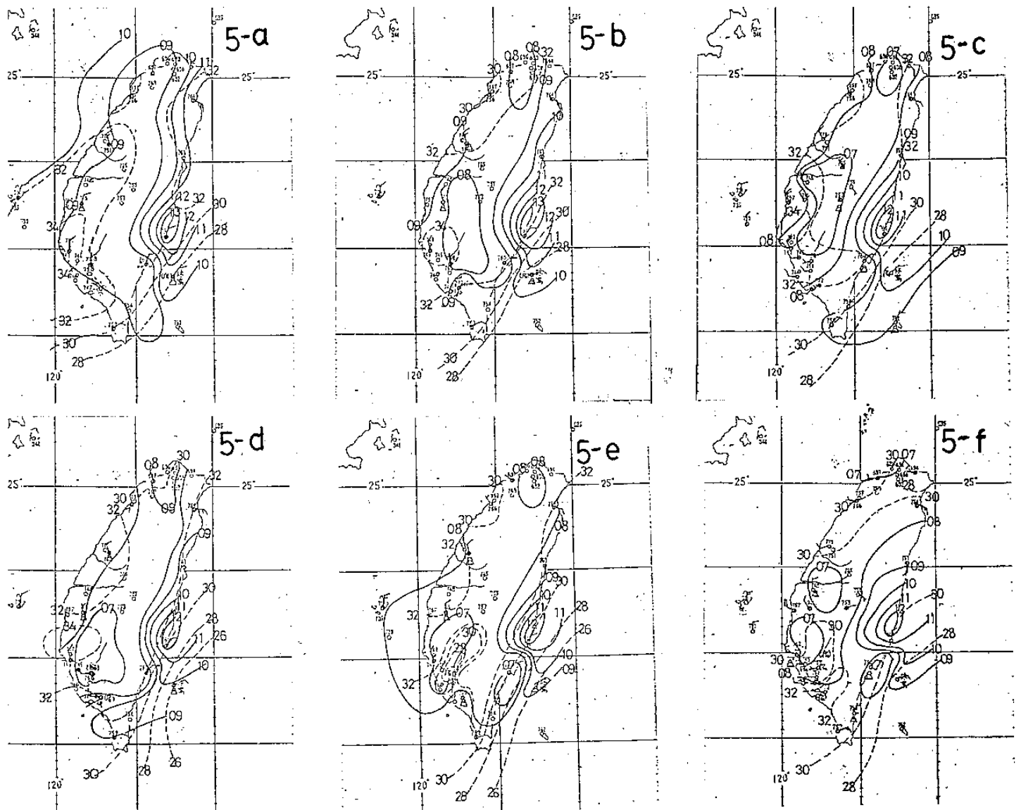
圖五：民國79年7月20日逐時(04Z~09Z；a~f)地面中尺度分析圖，實綫代表氣壓，虛綫代表溫度。
