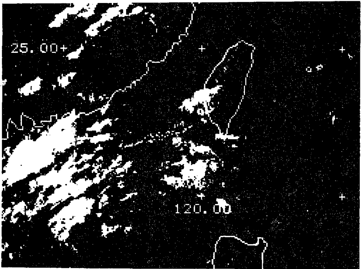
圖三：民國79年7月20日0933 Z，GMS-04可見光雲圖
