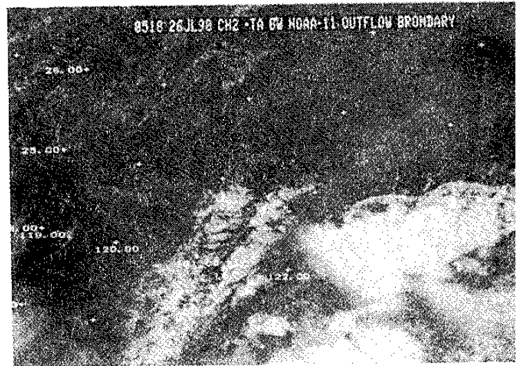
圖八：民國 79 年 7 月 26 日 0518 NOAA-11
