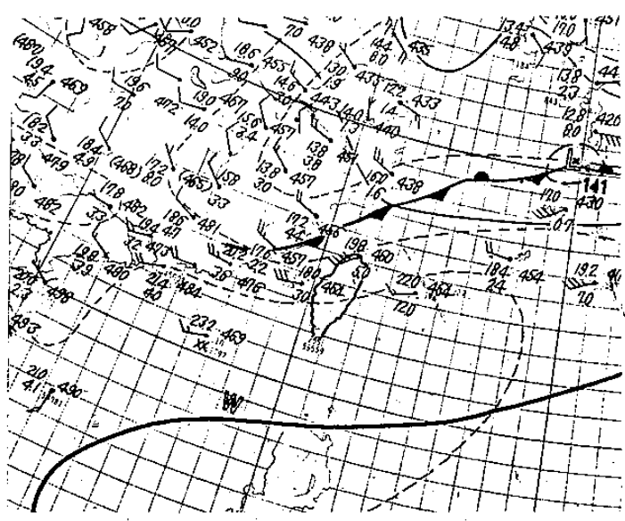
(b) 10月19日20L之850mb天氣圖
