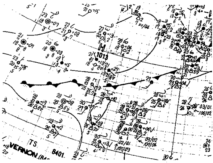
(a) 6月10日08L之地面圖
