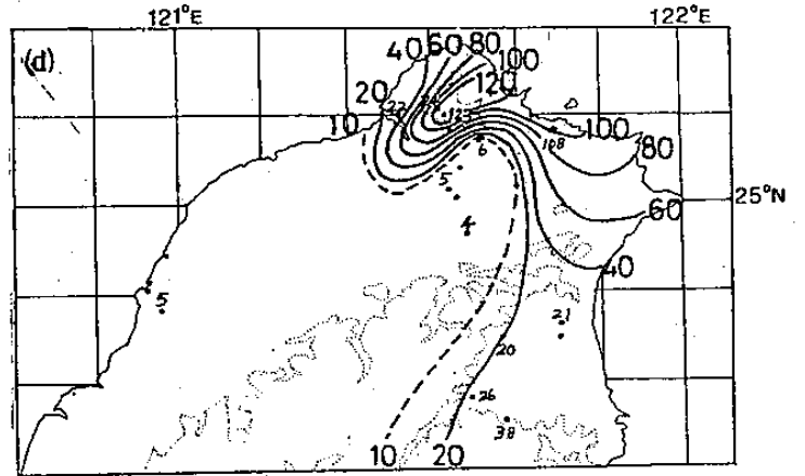
(d) 民 69 年 10 月 19 日 基隆 豪雨
