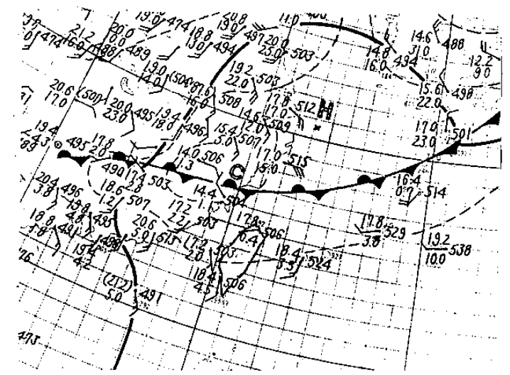
(b) 6月10日20L之850mb天氣圖
