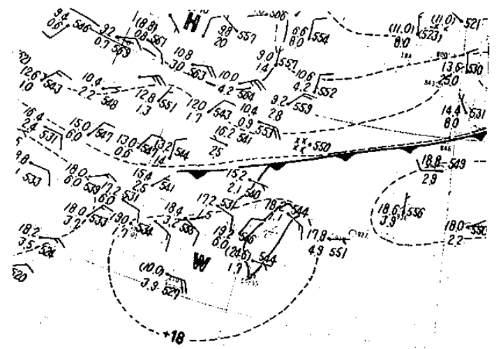
(b) 9月22日20L之850mb天氣圖
