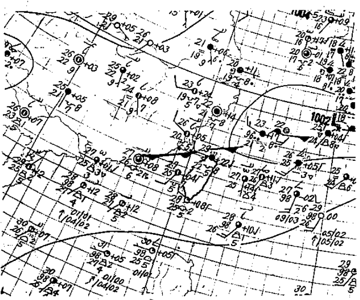
(a) 10月19日20L之地面天氣圖
