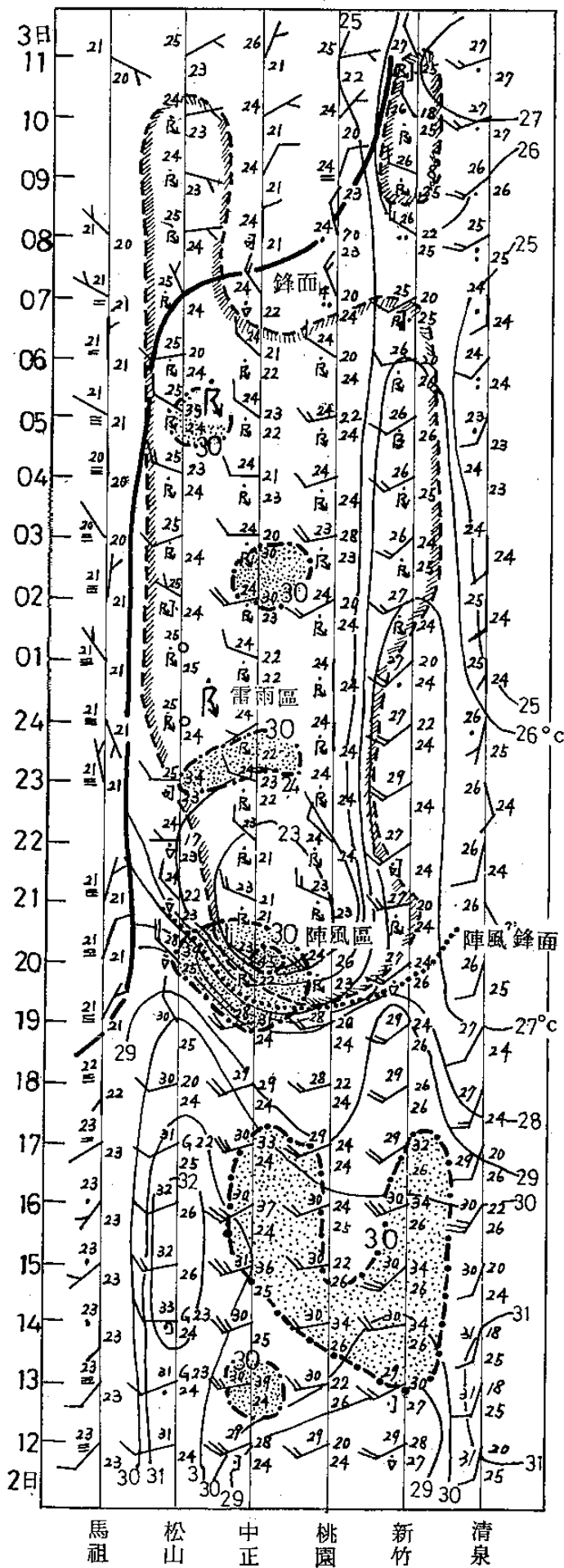
圖 8(a) 台北市 6·3 水災豪雨時(參見圖 10)。
