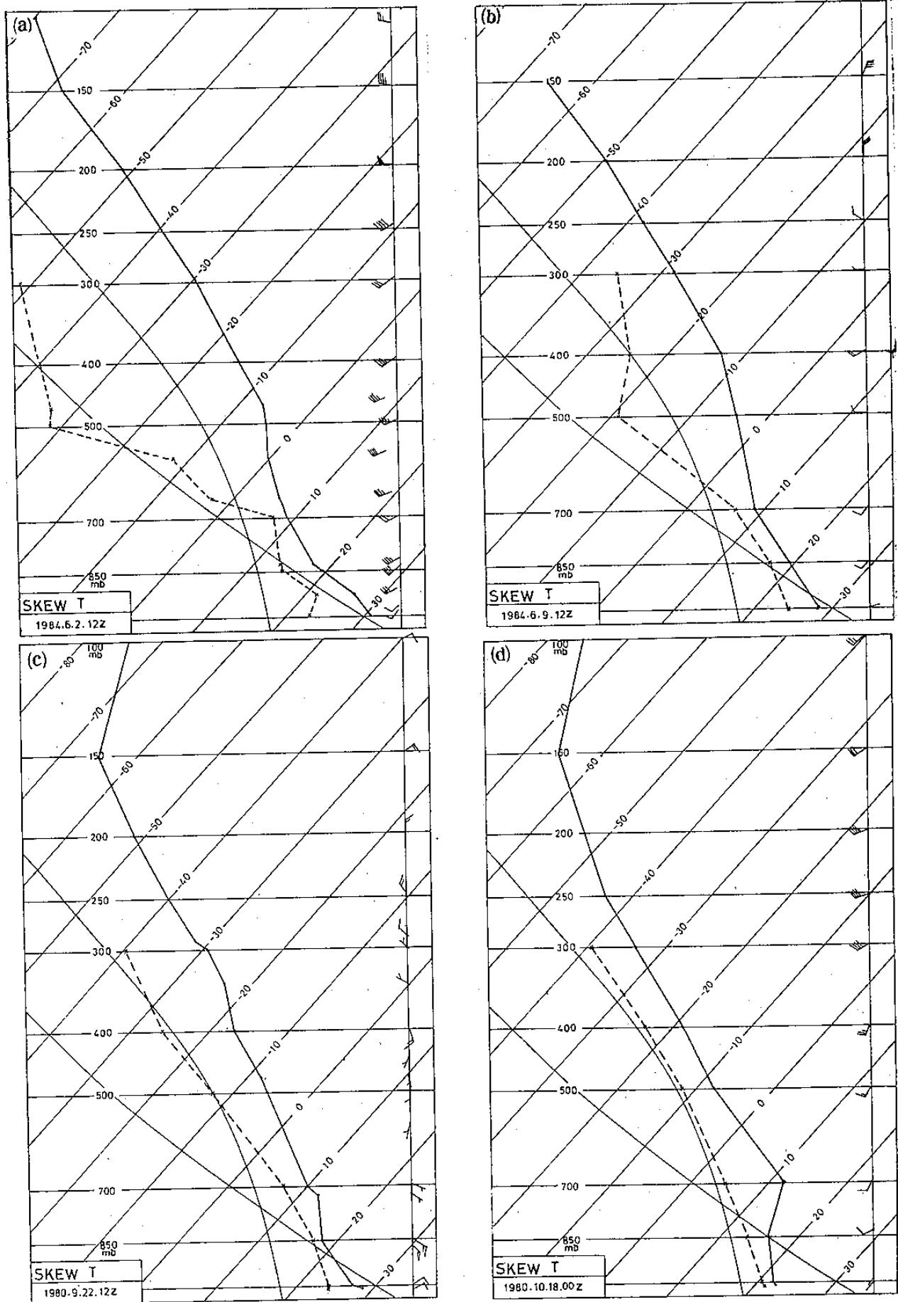
圖 16 四次豪雨期間前之台北氣團屬性。
