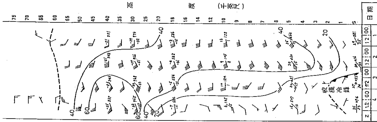
(a)民73年台北「6·3水災」豪雨 期間。
