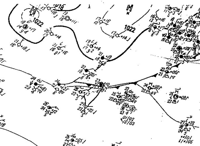
(a) 10月19日20L之地面圖
