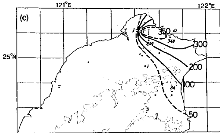
(c) 民 69 年 9 月 23 日 基隆 水災
