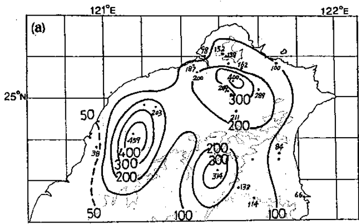
(a) 民 73 年 6 月 3 日 台北 水災
