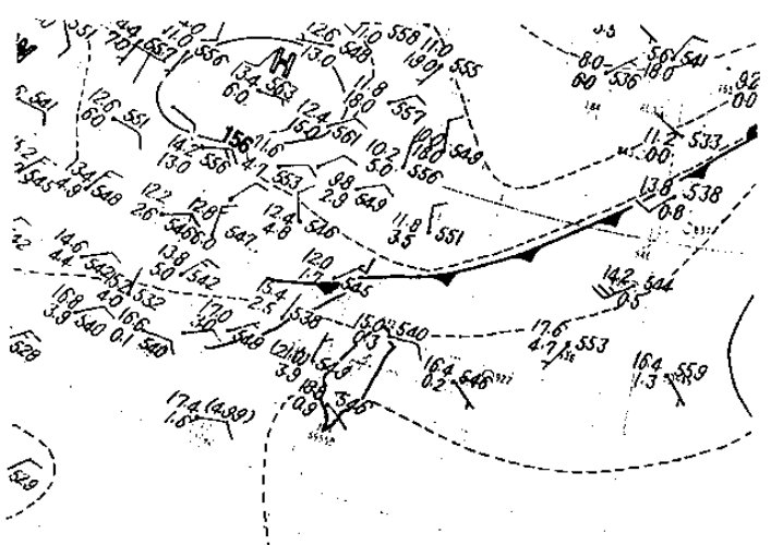
(b) 10月19日20L之850mb天氣圖
