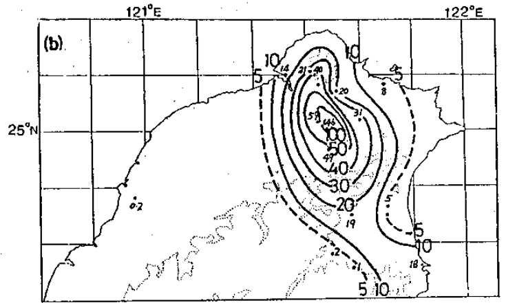
(b) 民 73 年 6 月 10 日 台北 水災
