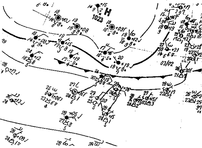
(a) 9月22日20L之地面圖
