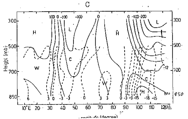
圖 6 : 1975 年 12 月 11 日歐亞大陸阻塞高壓重力位 高度及溫度之剖面圖。實線為高度 (m) 虛線為溫度 (°C)。 A : 65°N B : 55°N C : 45°N
