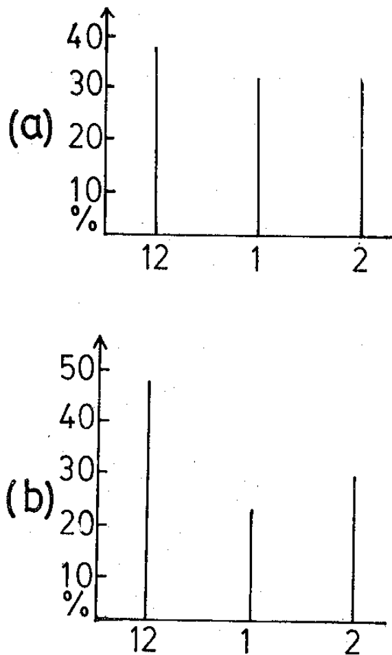
圖 4：阻塞高壓各月份發生次數百分率圖。
