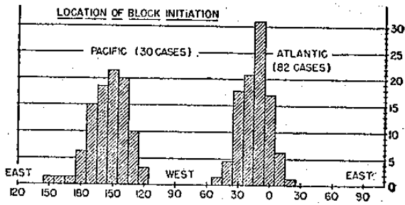
圖 3：各經度上阻塞高壓發生頻率圖
