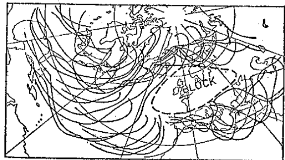
圖 2：阻塞後綜觀尺度系統移動圖。
