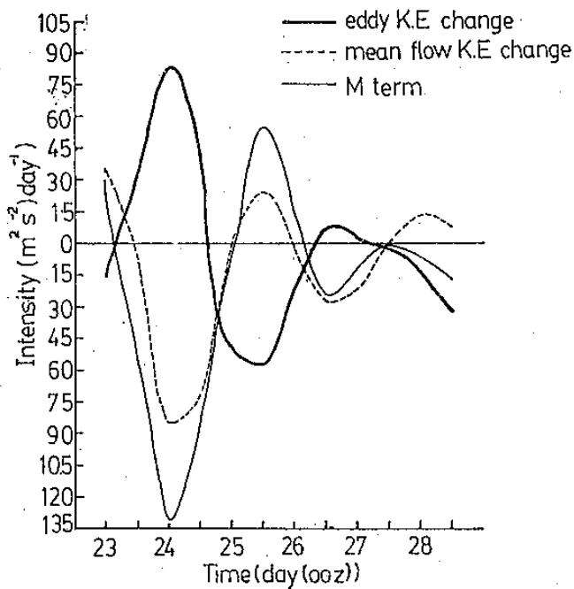
圖 13：太平洋阻塞高壓個案逐日能量變化圖 粗實綫為擾動動能，細實綫為正壓動能轉換量， 虛綫為平均氣流動能（1972年2月）。
