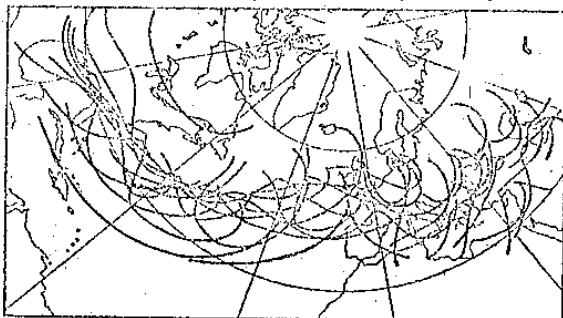
圖 1：阻塞前綜觀尺度系統移動圖。
