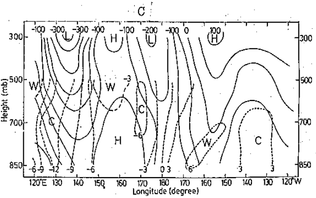
圖 9 : 1972 年 2 月 26 日太平洋阻塞高壓重力位 高度及溫度剖面圖。實綫為高度 ( m ) , 虛綫為溫度 ( °C ) 。 A : 65°N B : 55°N C : 45°N
