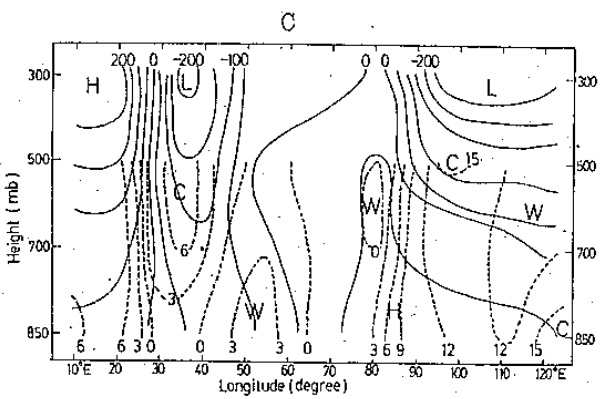
圖 5 : 1975 年 12 月 7 日歐亞大陸阻塞高壓重力位 高度及溫度之剖面圖。實線為高度 (m) 虛線為溫度 (°C)。 A 65°N B 55°N C 45°N
