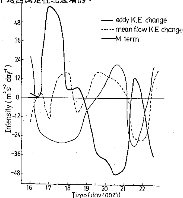
圖 12：歐亞大陸阻塞高壓個案逐日能量變化圖 粗實綫為擾動動能，細實綫為正壓動能轉換量， 虛綫為平均氣流動能 (1976年1月)。
