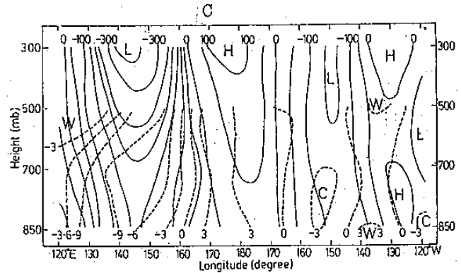
圖 10 : 1972 年 2 月 29 日太平洋阻塞高壓重力位 高度及溫度剖面圖。實綫為高度 ( m ) , 虛綫為溫度 ( °C ) 。 A : 65°N B : 55°N C : 45°N
