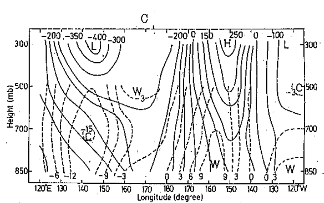
圖 8 : 1972 年 2 月 23 日 太平洋阻塞高壓重力位 高度及溫度剖面圖。實綫為高度 ( m ) , 虛綫為溫度 ( °C ) .
