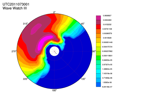
圖 13 方向波譜圖範例
