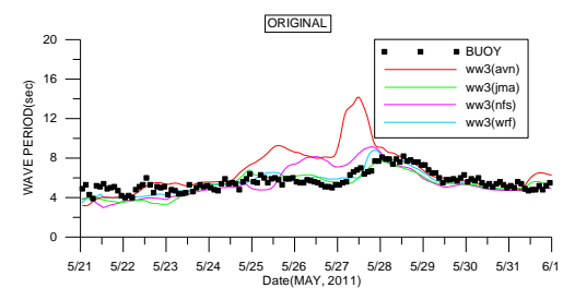
圖6 修正前的周期與實測周期比較時序列圖
